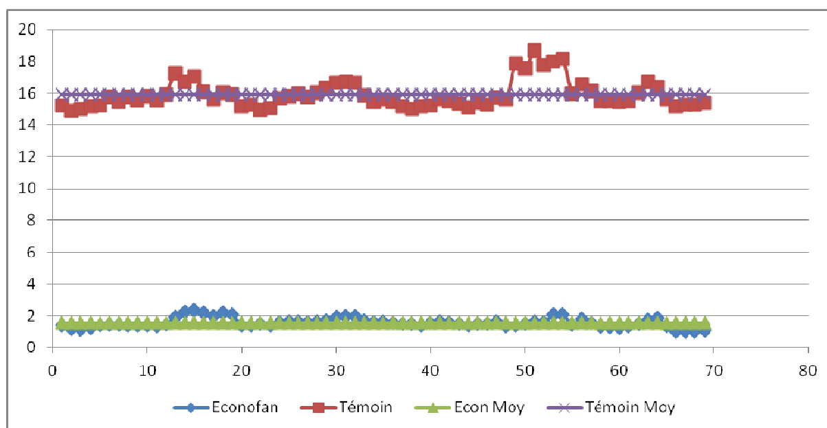
Graphique 1 : Consommation du ventilateur EconoFan vs Témoin
